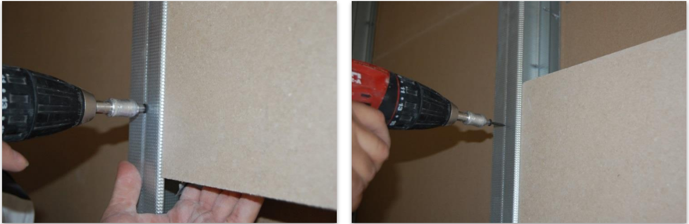
Bild 4: Fixierung der Rigips Traverse im offenen Profil
